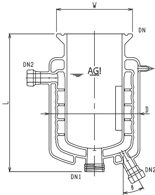
媒体バッフル付三重管式反応容器 (3972) (図面は攪拌バッフル付です)
