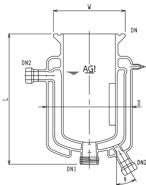
三重管式反応容器 (3970) (図面は攪拌バッフル付です)
